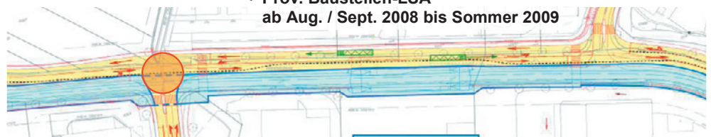
Abbildung 13: Provisorische Baustellen-LSA am Knoten Hertistrasse / Weststrasse
